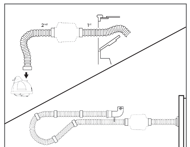
4 Instale el colador / Hayward Vac Lock®
